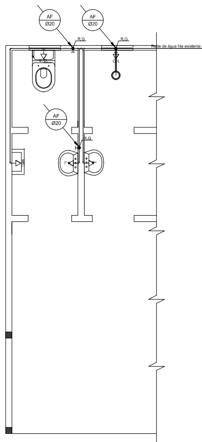
PROJETO HIDRÁULICO ESC. 1/50
