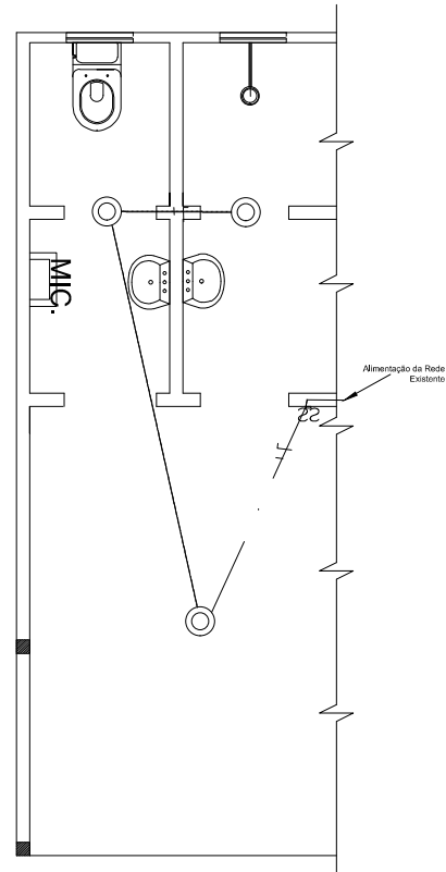
ELÉTRICO ESC. 1/50
