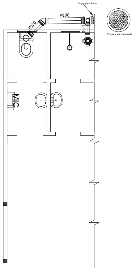
PROJETO ESGOTO ESC. 1/50
