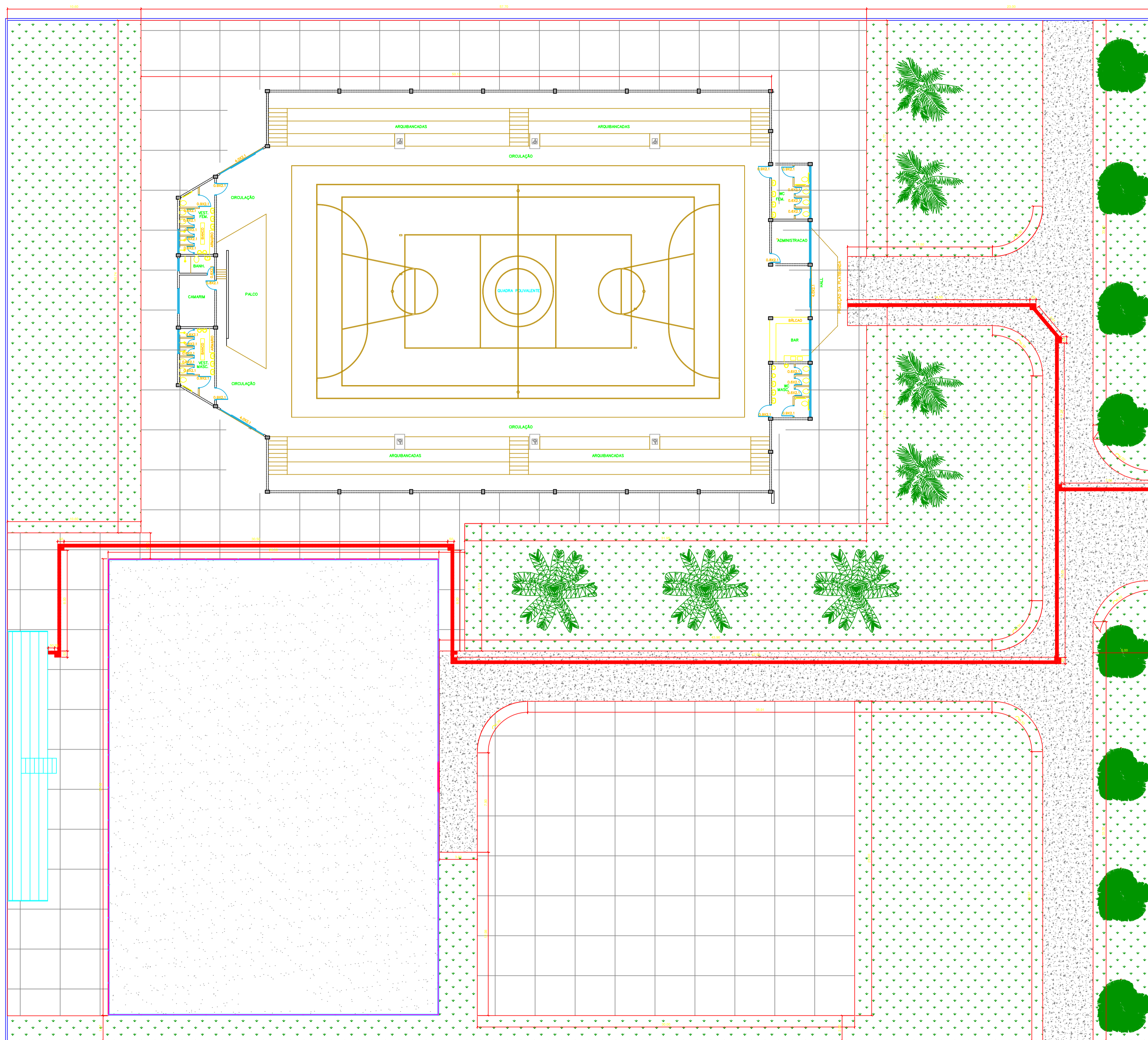
PLANTA BAIXA - COMPLEXO POLIESPORTIVO ESC: 1/100
